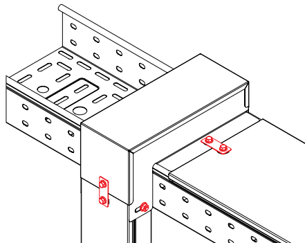
Вертикальный отвод эксплуатируемой кабельной трассы (не требует распиливания лотков) с использованием ответвитель-крышки DDS
