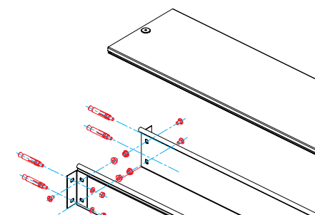
Ввод кабельной трассы в стену или оборудование (щит, шкаф и др.) с использованием опорных уголков FR
