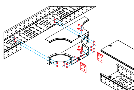
Изменение уровня прокладки кабельной трассы (соединение шарнирного типа) с использованием соединительных пластин GSV и защитных пластин RP
