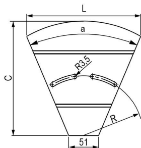
Чертеж основания
