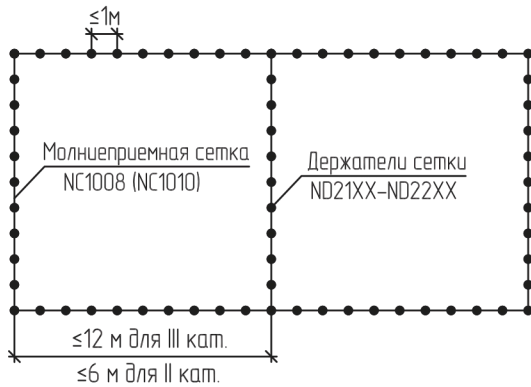
Рис. 2 Эскиз молниеприемной сетки на крыше здания
