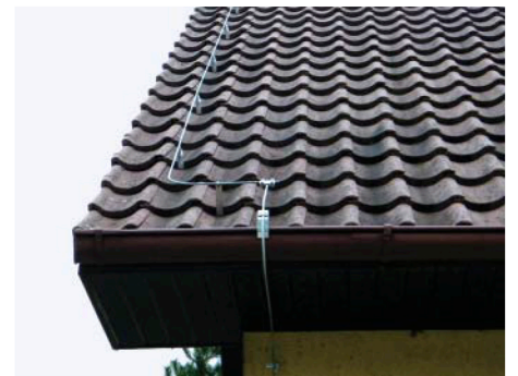
Токоотвод, смонтированный на черепичной кровле
